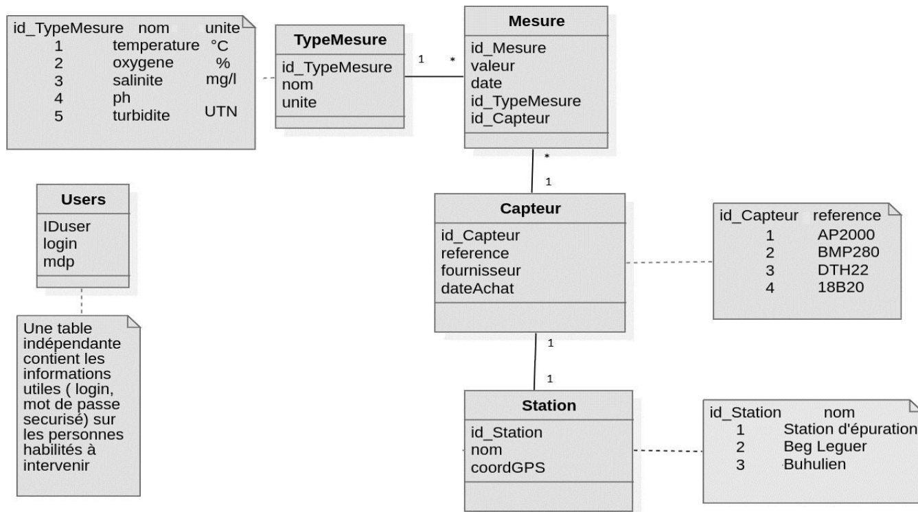
Figure 6 : Structure de la base de données
