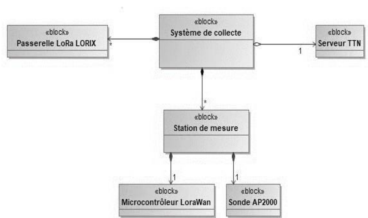
Figure 2: Diagramme de blocs du système de collecte
